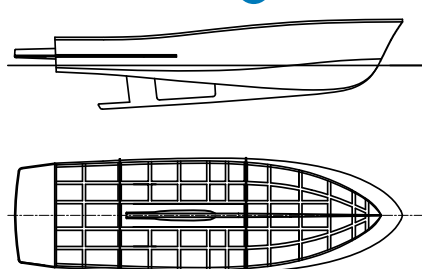
Kadłub SKEIRON INBOARD E
