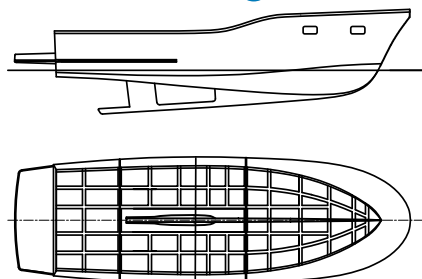
Kadłub SKEIRON INBOARD B
