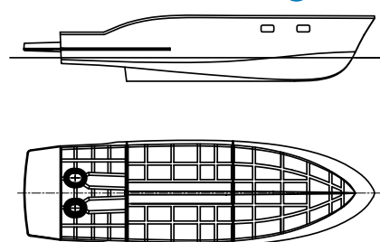
Kadłub SKEIRON IPS/STERNDRIVE D
