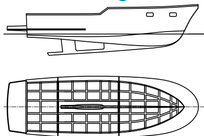
Kadłub SKEIRON INBOARD A
