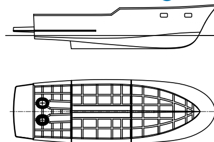
Kadłub SKEIRON IPS/STERNDRIVE A
