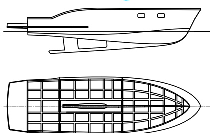
Kadłub SKEIRON INBOARD D
