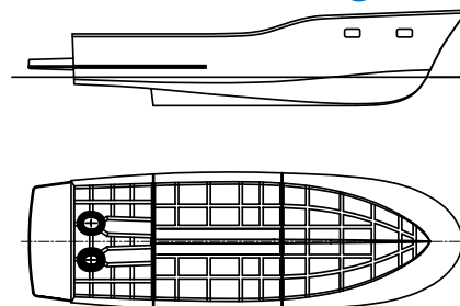
Kadłub SKEIRON IPS/STERNDRIVE B
